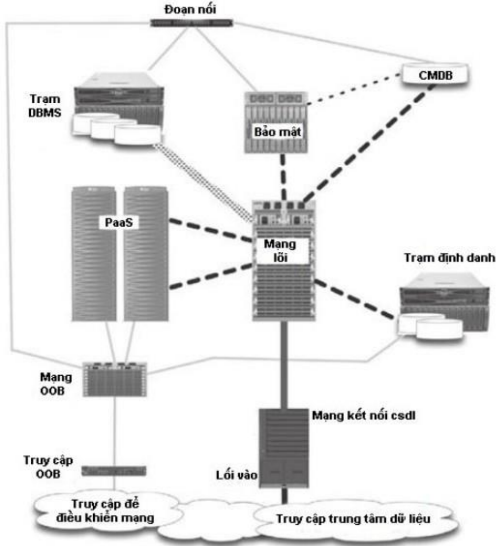
Hình 4.4. Kiến trúc đám mây cung cấp dịch vụ định danh và dịch vụ cơ sở dữ liệu Kiến trúc đám mây cung cấp kho lưu trữ và dịch vụ tính toán
