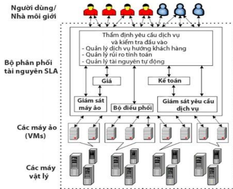
Hình 2.10. Kiến trúc Market-Oriented Cloud
