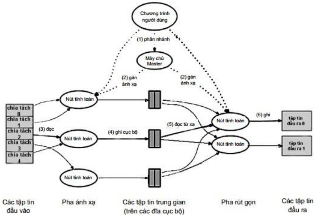
Hình 3.6. Mô tả quá trình thực thi gói công việc
