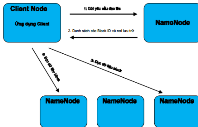
Hình 3.3. Quá trình đọc tập tin trên HDFS
