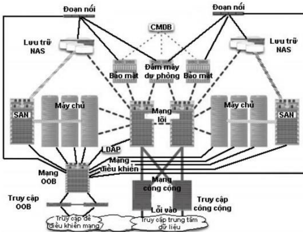
Hình 4.5. Kiến trúc đám mây cung cấp dịch vụ tính toán và lưu trữ
