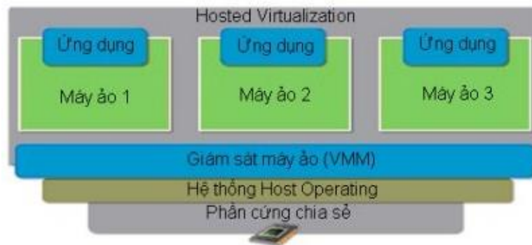
Hình 2.4. Mô hình ảo hóa Hosted-based
