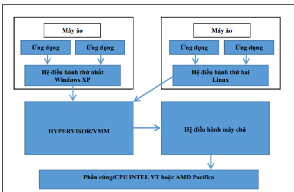
Hình 2.6. Kiến trúc ảo hóa Hybrid
