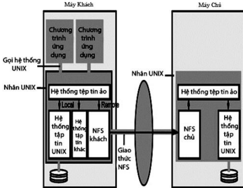
Hình 3.1. Kiến trúc hệ thống tệp tin NFS
