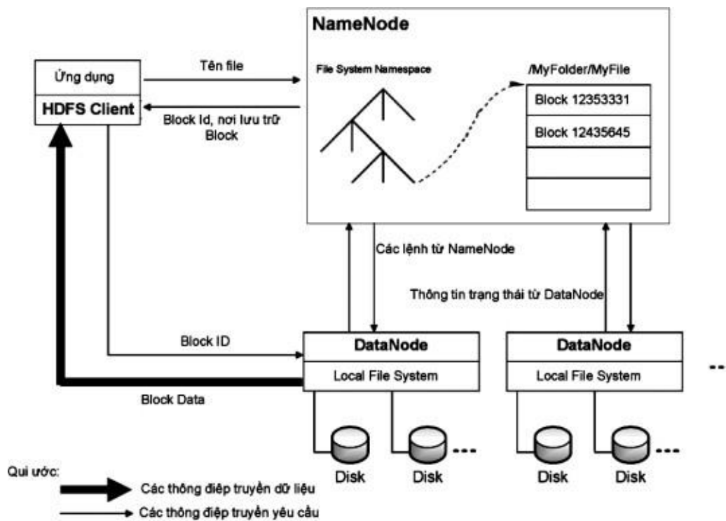
Hình 3.2. Kiến trúc HDFS
