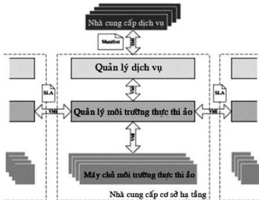
Hình 6.1. Kiến trúc RESERVOIR: Các thành phần và giao diện chính
