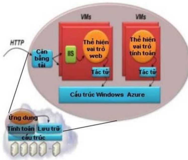
Hình 5.5. Windows Azure cung cấp các dịch vụ lưu trữ và tính toán cho đám mây
