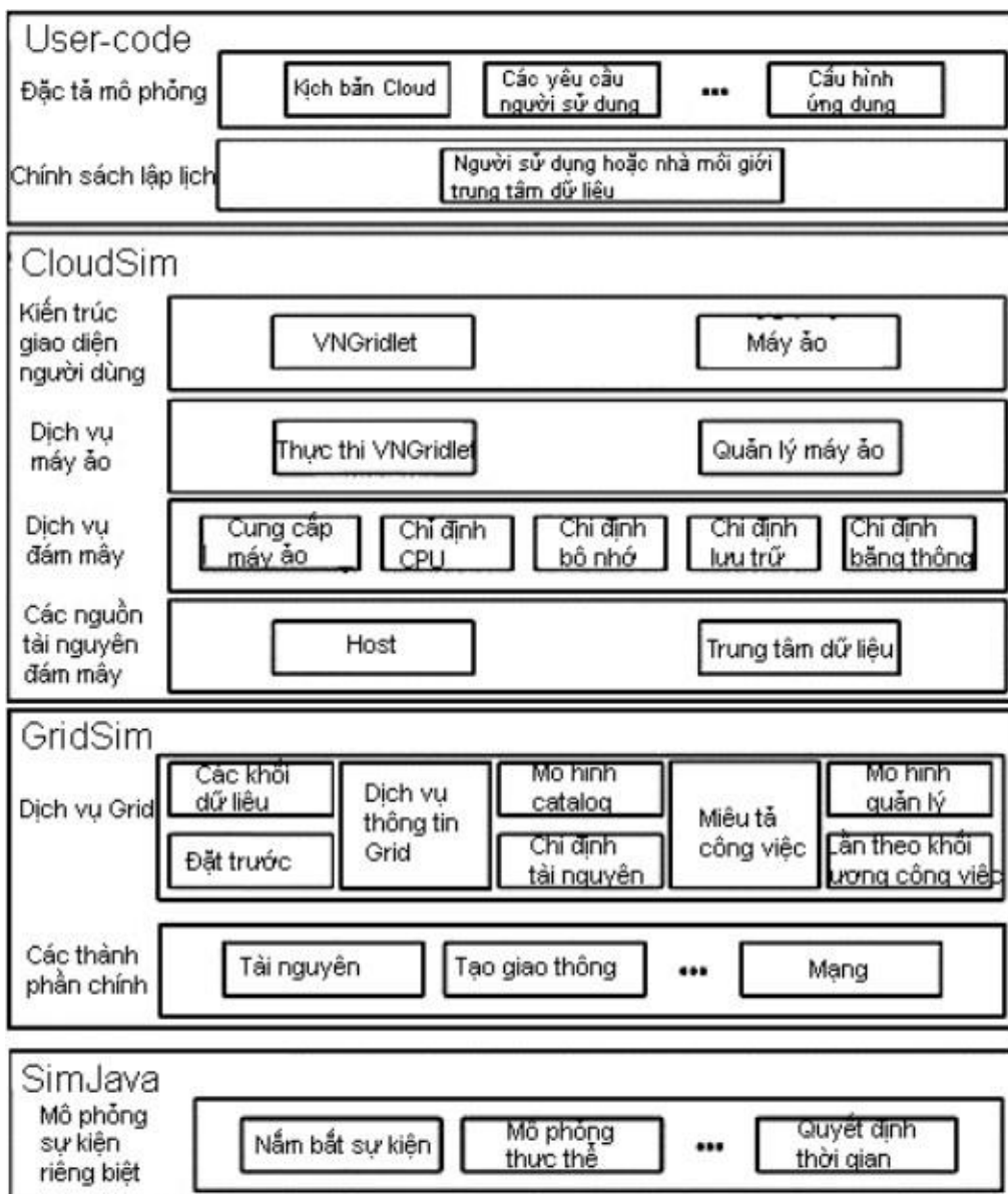
Hình 2.11. Kiến trúc lớp của CloudSim
