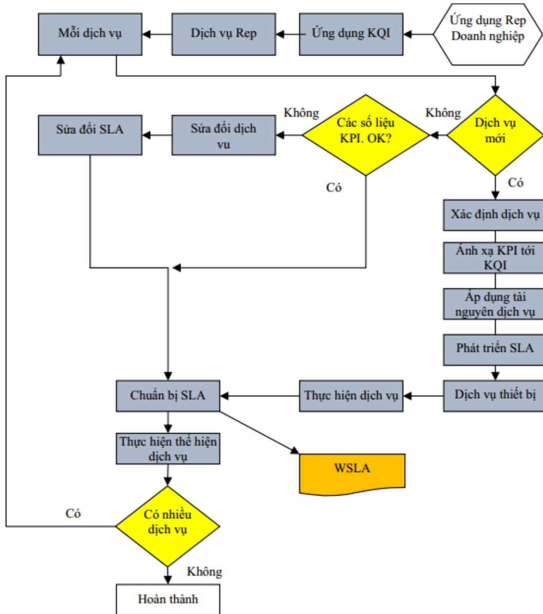
Hình 6.6. Quy trình xây dựng SLA
