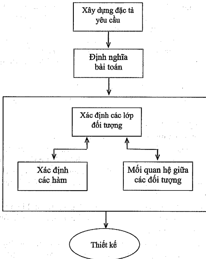
Hình 1-2. Sơ đồ các bước phân tích hướng đối tượng
