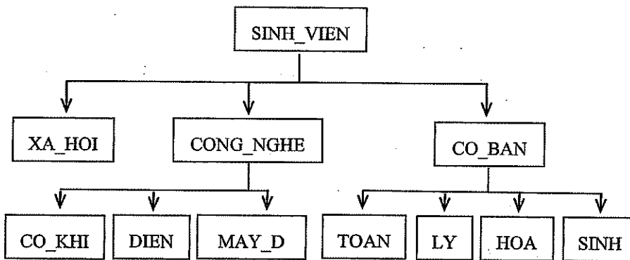
Hình 3.4. Cấu trúc phân cấp các lớp trong quan hệ kế thừa
