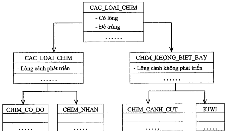
Hình 2-1. Quan hệ kế thừa
