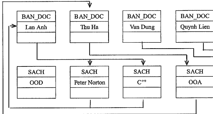
Hình 1-10. Thể hiện mối quan hệ giữa hai lớp đối tượng SACH và BAN_DOC
