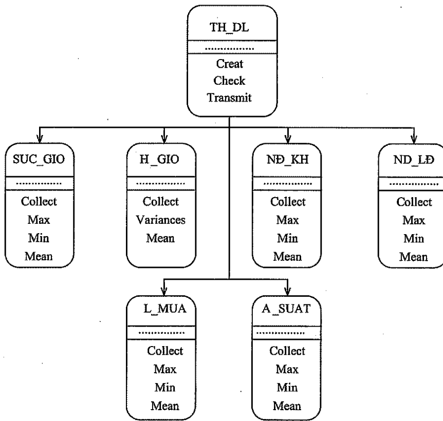
Hình 2-7. Mô tả quan hệ của các lớp đối tượng "mềm"
