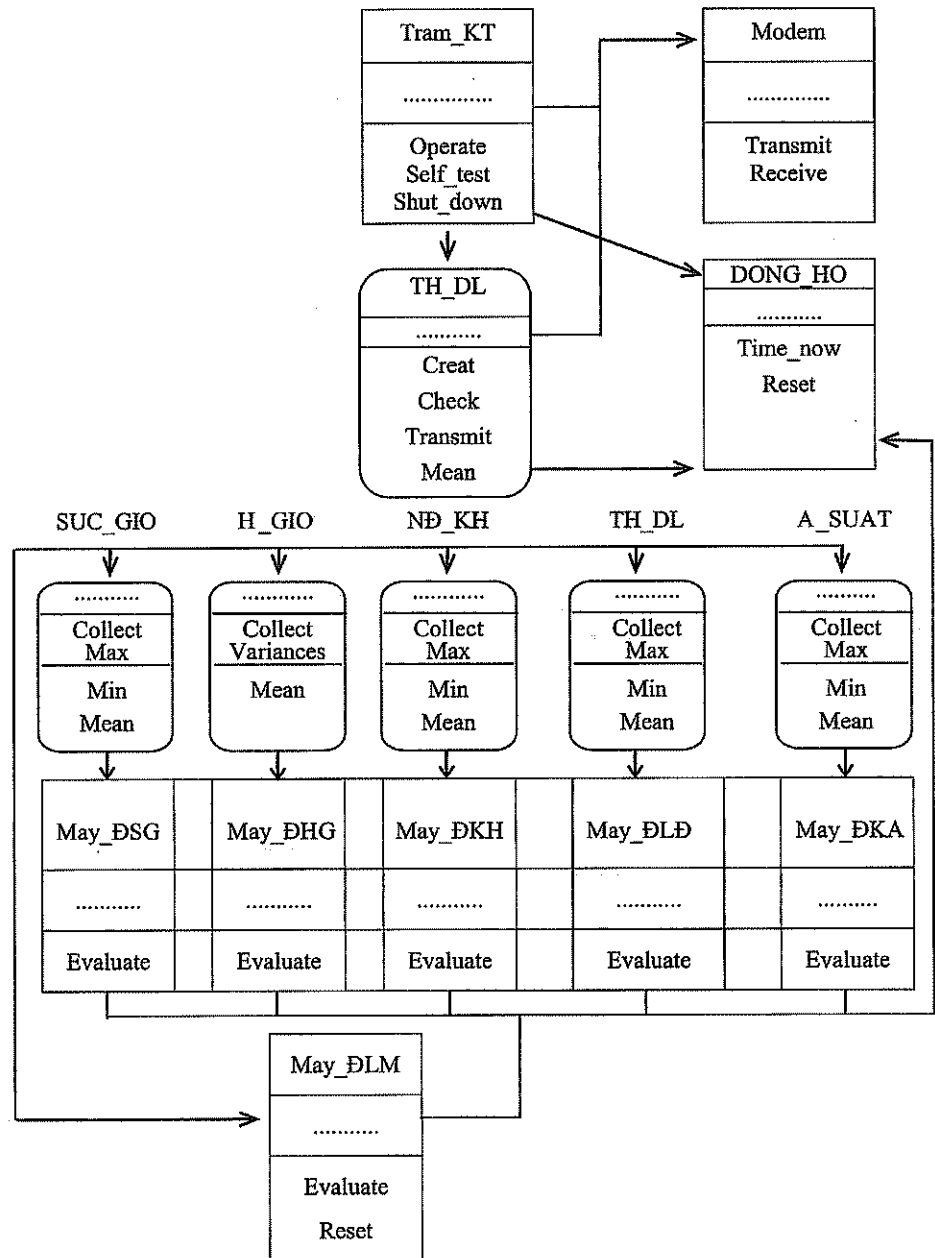
Hình 2-8. Cấu trúc hệ thống khí tượng thủy văn
