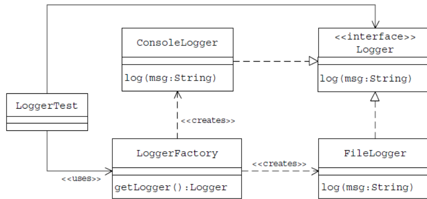
Hình 8.4: LoggerTest truy nhập với LoggerFactory
