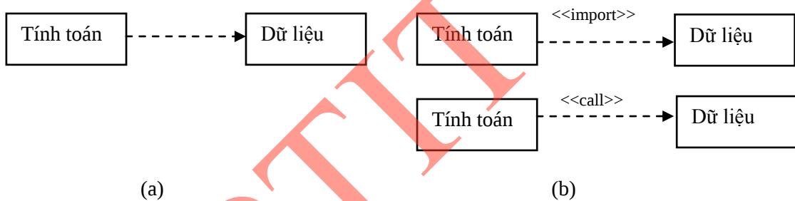
Hình 3.2: (a) Biểu diễn phụ thuộc (b) Sử dụng nhãn để thể hiện ngữ nghĩa
