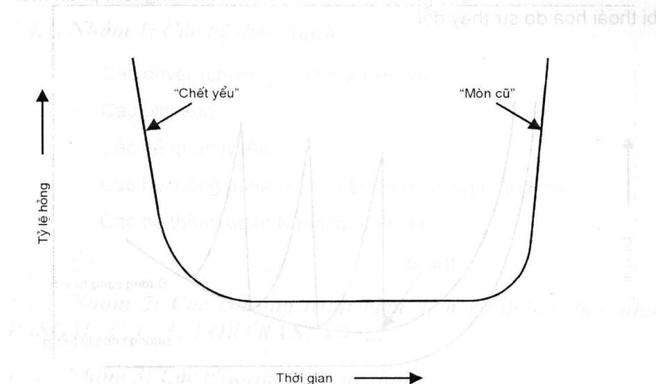
H 1.1. Đường cong hỏng hóc cho phần cứng
