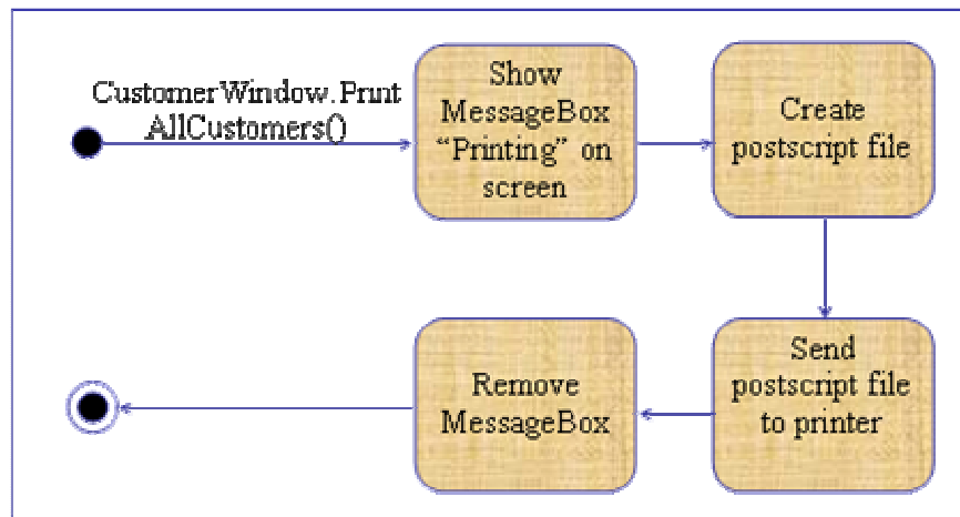
Hình 19.8. Khi một người gọi tác vụ PrintAllCustomer (trong lớp CustomerWindow ), các hành động khởi động. hành động đầu tiên là hiện một hộp thông báo lên màn hình; hành động thứ hai là tạo một tập tin postscript; hành động thứ ba là gửi file postscript đến máy in; và hành động thứ tư là xóa hộp thông báo trên màn hình. Các hành động được chuyển tiếp tự động; chúng xảy ra ngay khi hành động trong giai đoạn nguồn được thực hiện.
