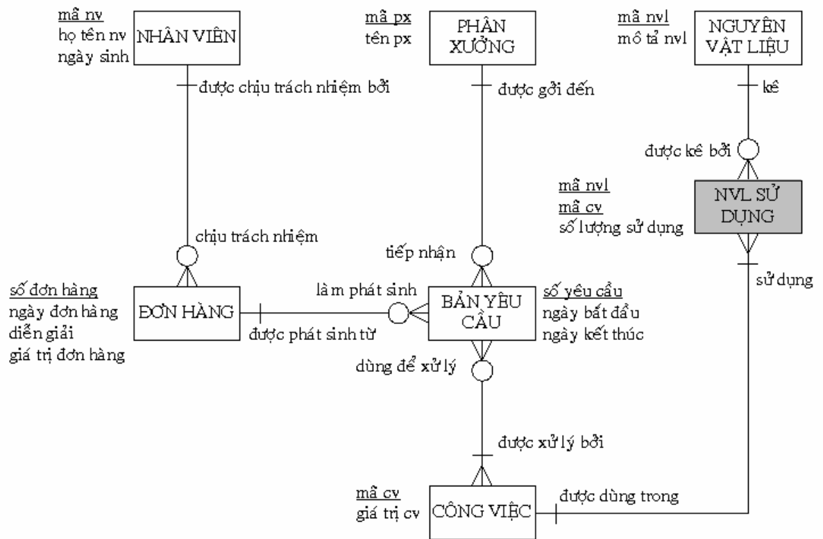
Hình 6-5 Biểu đồ quan hệ dữ liệu của hệ thống quản lý phân xưởng
