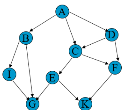
Đồ thị không gian trạng thái
