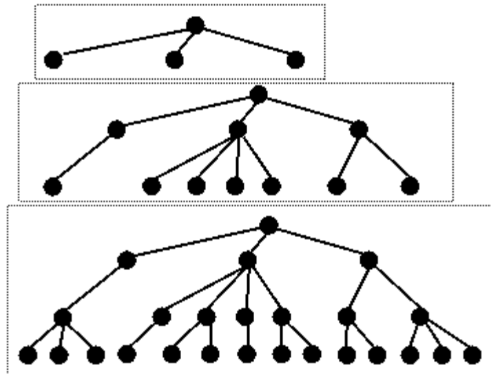
Hình 2.10: Tìm kiếm theo chiều rộng
