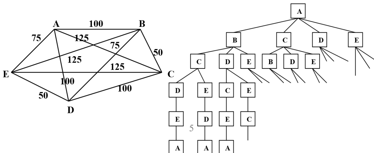
Hình 2.8: Ví dụ bài toán hành trình người bán hàng và một phần không gian trạng thái
