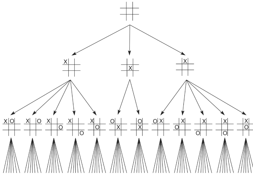
Hình 2.2: Một phần không gian trạng thái của trò chơi Tic-tac-toe
