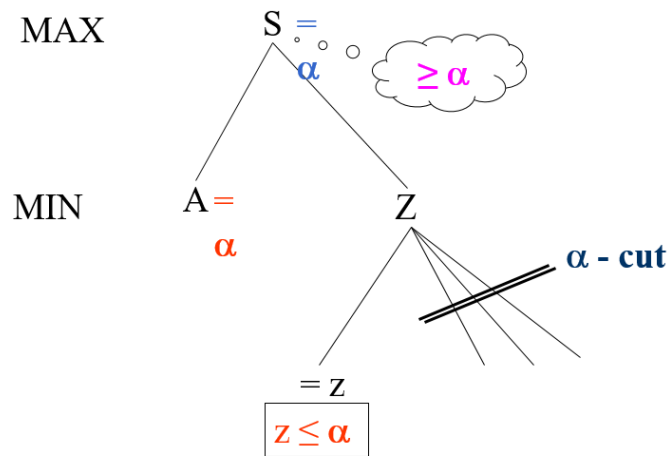
Hình: Cắt tia \alpha
