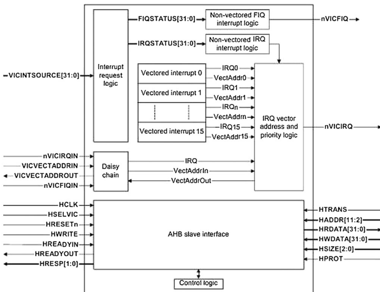
Fig. 3.1 ARM PL190 VIC
